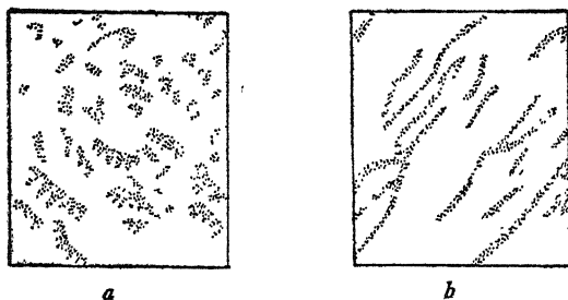
चित्र १९७—भारतीय मरुस्थल में रेत की पहाड़ियाँ
